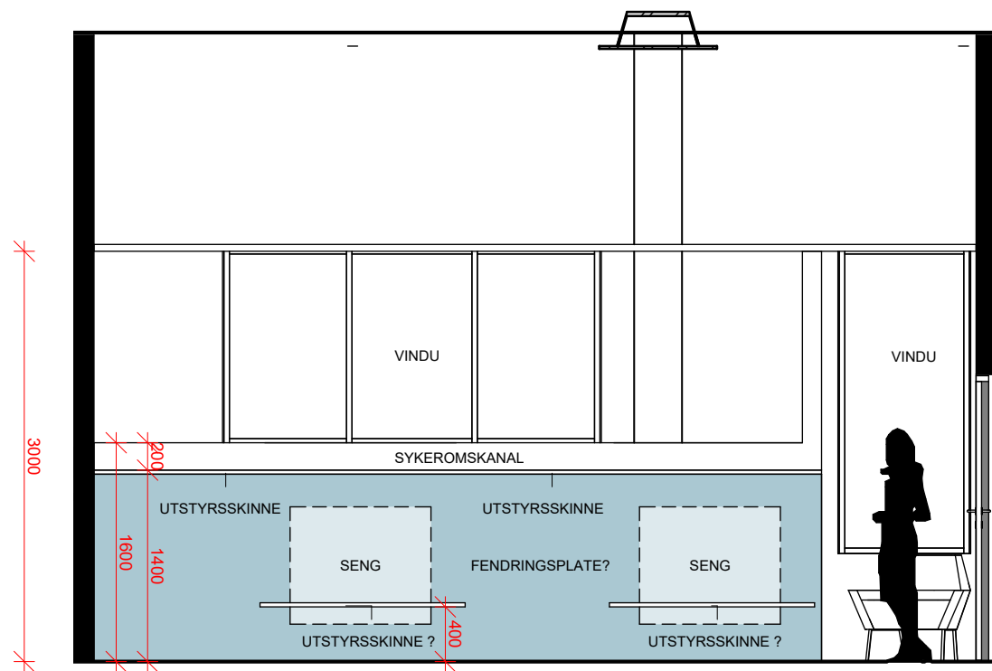
Oppriss 2-sengsrom_horizontal kanal
