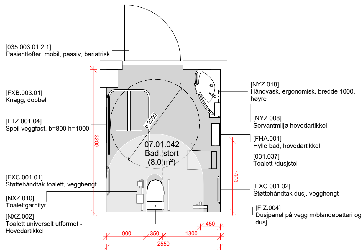
Planutsnitt 07.01.042 Bad, stort
